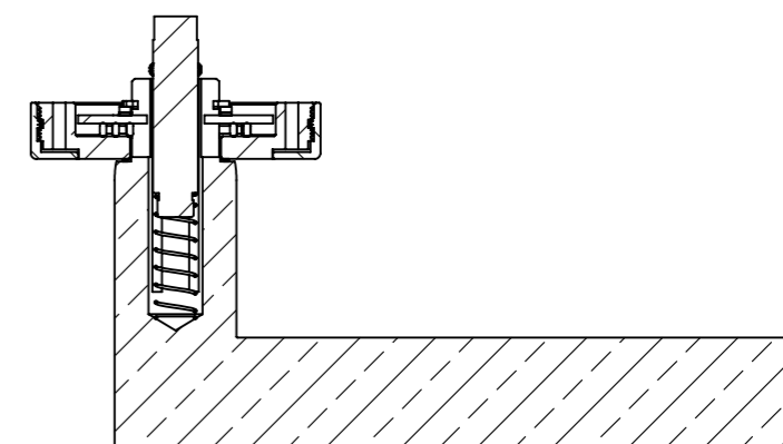
SECTION D-D
