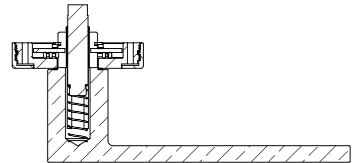
SECTION D-D
