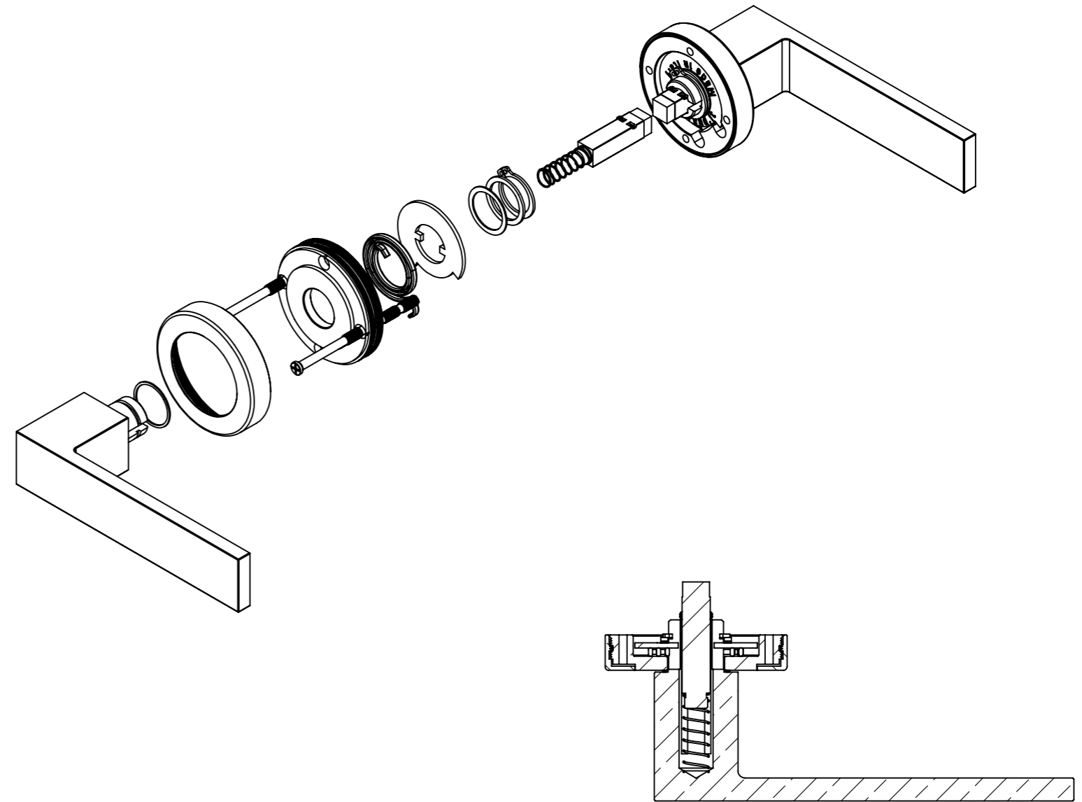
SECTION D-D
